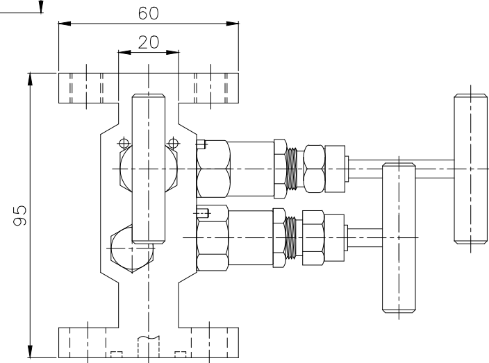
VIEW:- 'BB'
